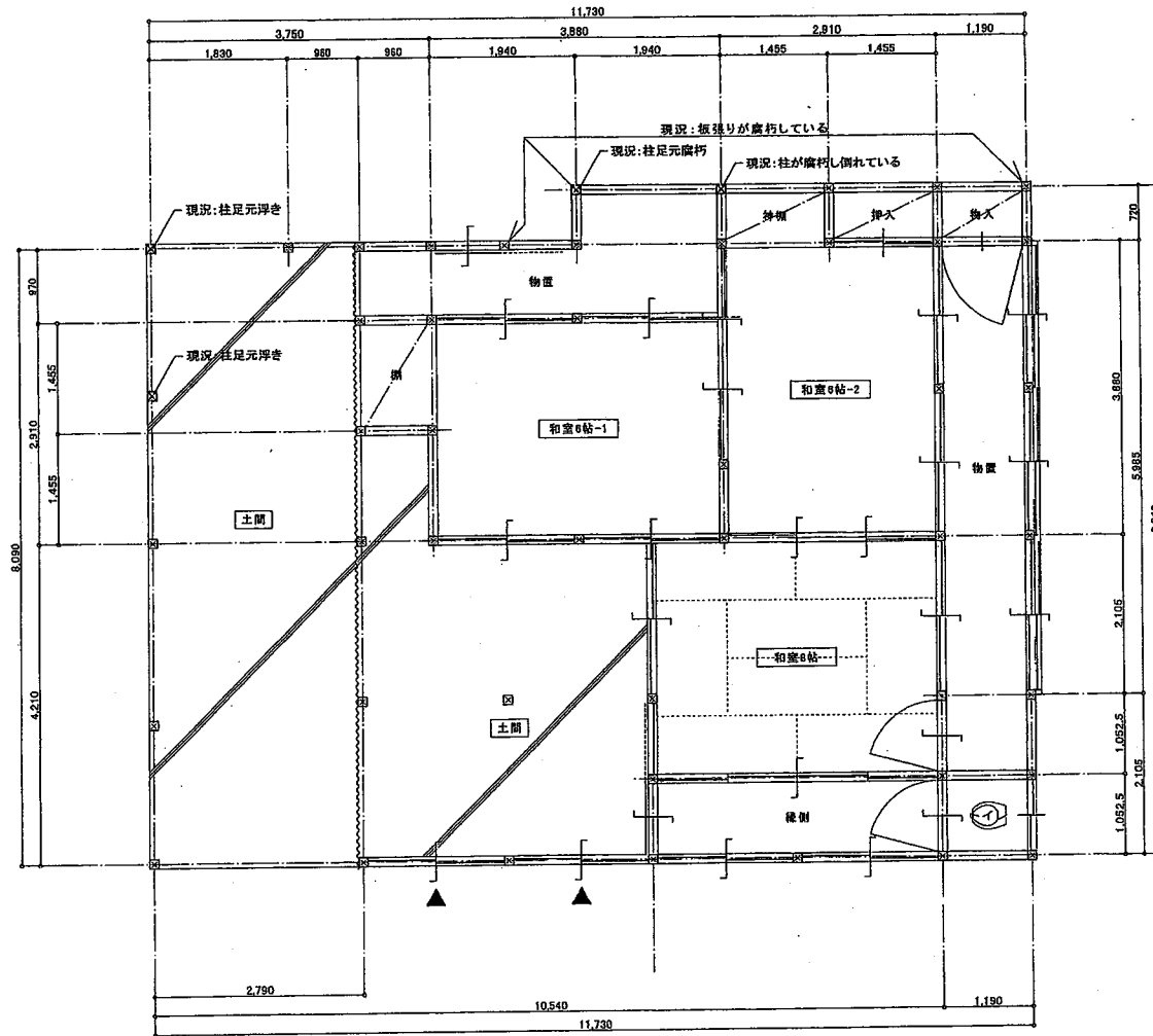
現況平面図 S = 1 / 50
