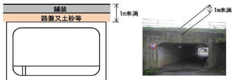
図 11 溝橋(ボックスカルバート)の考え方
